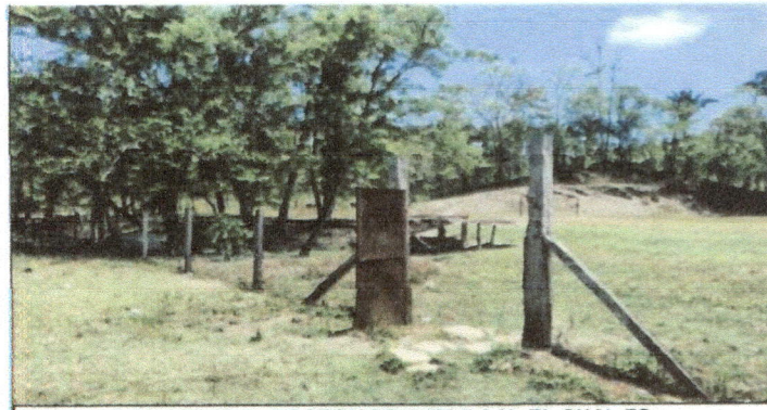
Foto 6: SE OBSERVA EL PORTON DE 1.5M X 2 M, EL CUAL ES NECESARIO SUSTITUIR COLUMNAS DE MADERA A CONCRETO.
