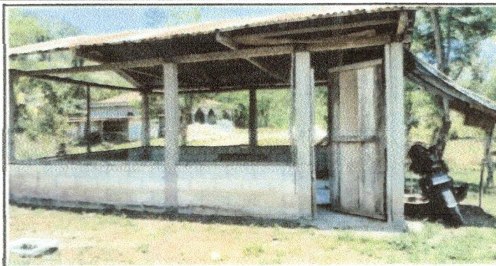
Foto 1: MEJORAMIENTO DE COCINA REPARACIÓN DE COLUMNAS SUSTITUCIÓN DE MADERA POR BLOCK Y SUSTITUCIÓN DE MALLA POR BALCONES DE METAL Y SUSTITUCIÓN DE PUERTA DE MADERA POR METAL.
